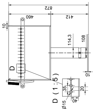
Ansicht ( 1:10 )
