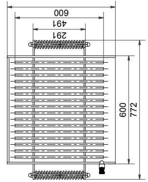
Grundriss
